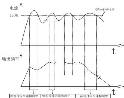
过流失速动作示意图
