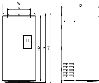
55~250kW 尺寸图 (含 132~250kW 的标准机)
