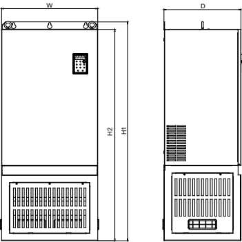
132~250kW 非标机（有底座）
