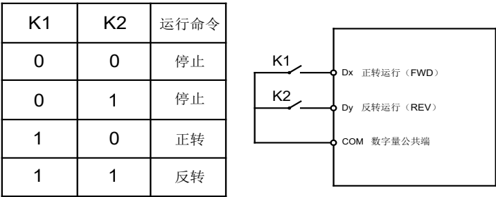
图 6-6 两线式模式 2
