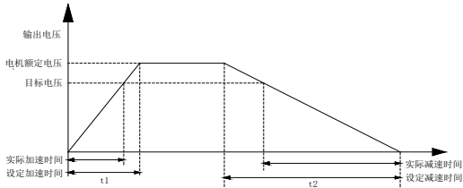
V/F 分离示意图
