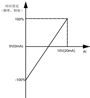
图 6-9 模拟给定与设定量的对应关系
