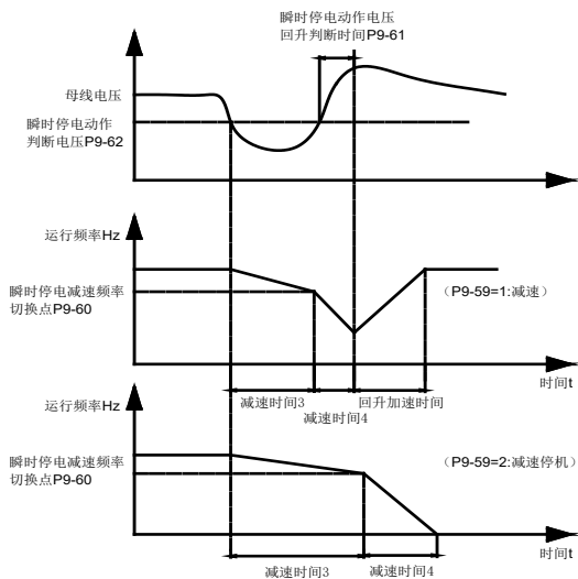
图 6-23 瞬时停电动作示意图
