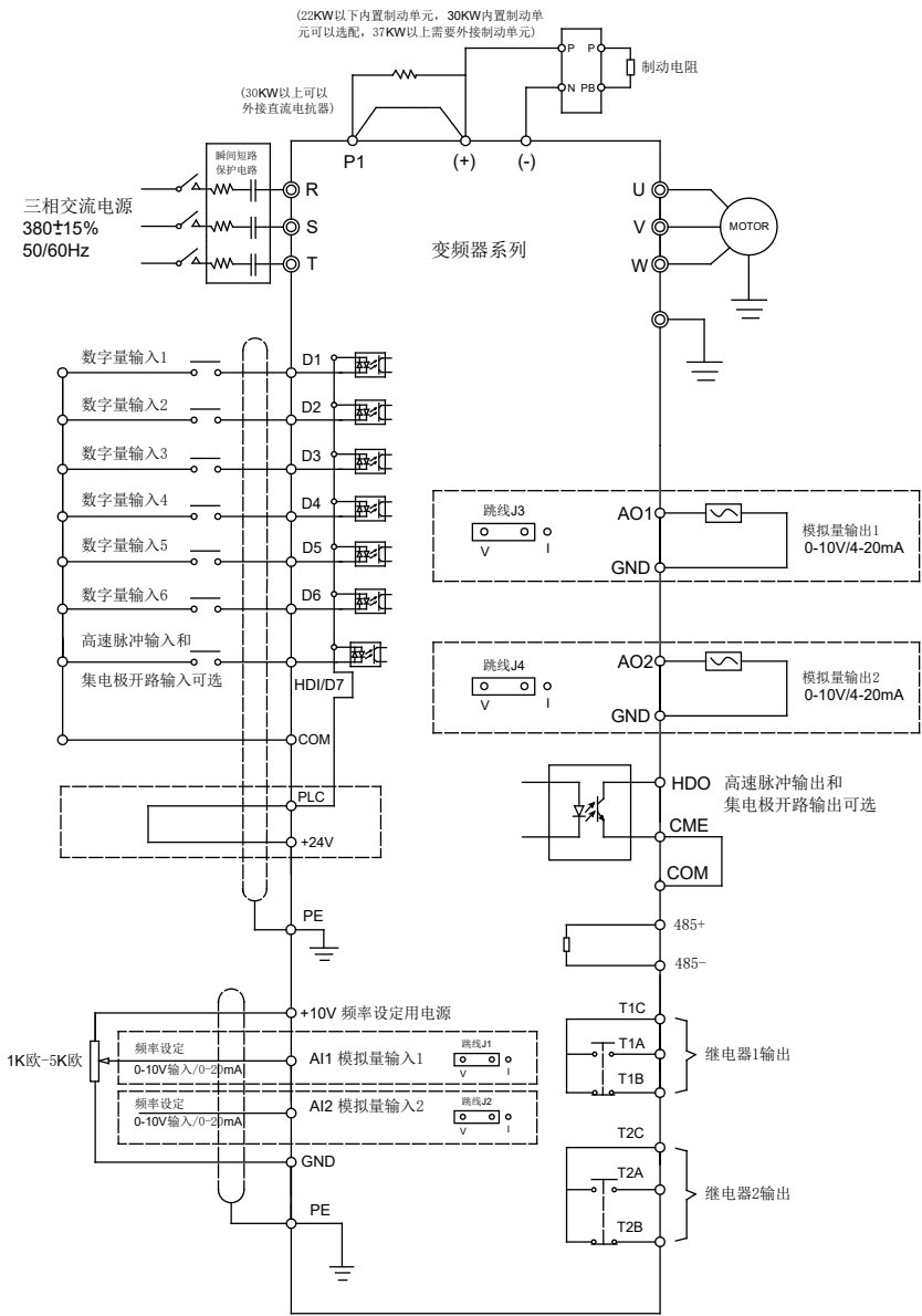
图 3-4 其它功率变频器接线图
