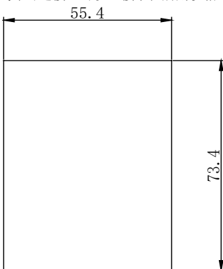
应用此键盘外引时机箱开孔尺寸
