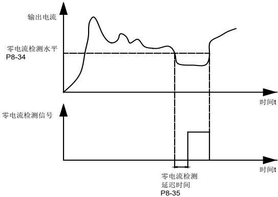
图 6-20 零电流检测示意图
