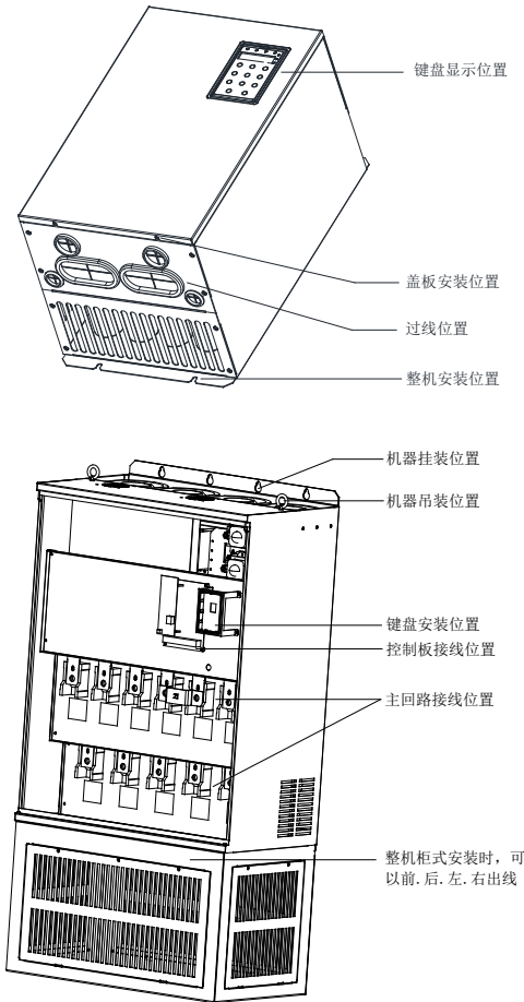
图 2-3 变频器各部件说明
