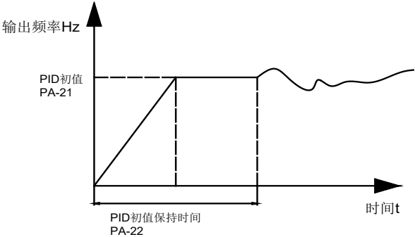
图 6-26 PID 初值功能示意图
