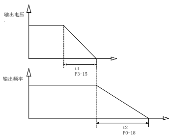
V/F 分离频率/电压先后下降示意图
