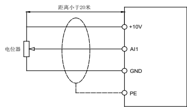
图 3-15 模拟量输入端子接线示意图
