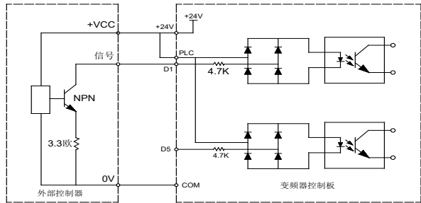
图 3-17 漏型接线方法
