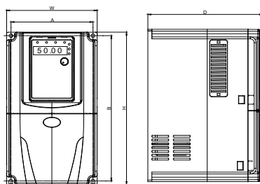
0.75~11kW 尺寸图
