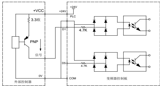
图 3-18 源型接线方法
