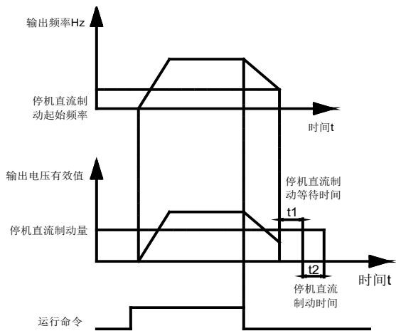
图 6-12 停机直流制动示意图
