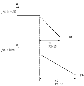
V/F 分离输出电压/频率独立减至 0
