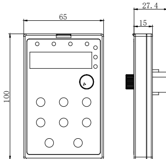
其它功率变频器用 65*100mm 键盘尺寸
