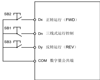
图 6-7 三线式控制模式 1
