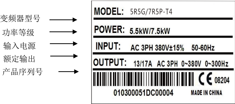
图 2-2 铭牌说明
