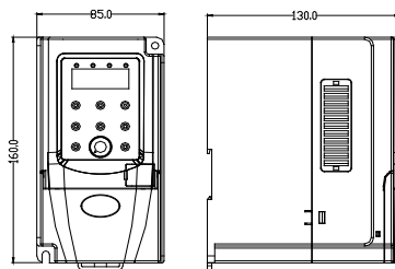
X 系列 0.75~4kW 尺寸图(单管机器)
