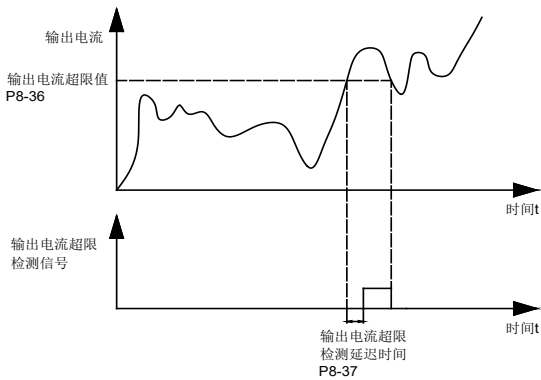
图 6-21 输出电流超限功能示意图
