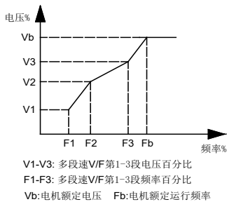
图 6-4 多点 V/F 曲线设定示意图
