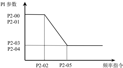
图6-2 PI参数示意图
