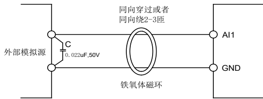
图 3-16 模拟量输入端子处理接线图
