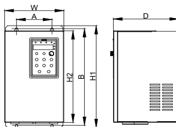
15~45kW 尺寸图
