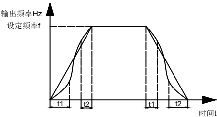
图 6-10 S 曲线加减速 A 示意图
