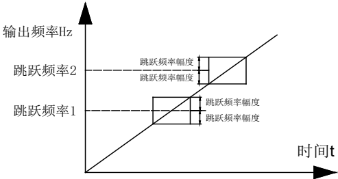
图 6-13 跳跃频率示意图
