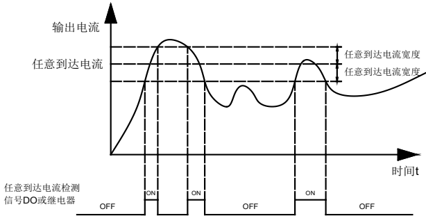
图 6-22 任意到达电流检测示意图
