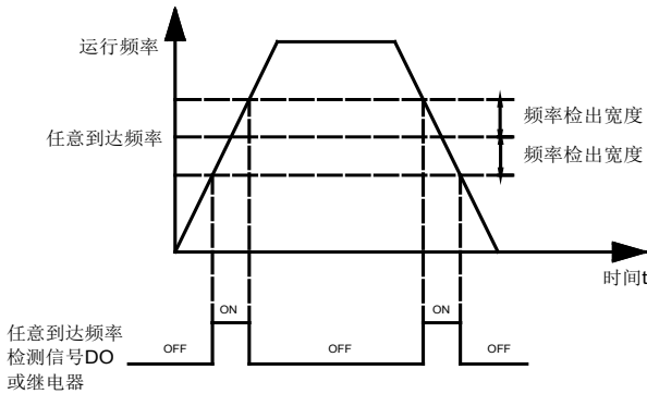
图 6-19 任意到达频率检测示意图
