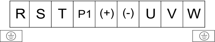
图 3-11 主回路端子图（三相 380V，37~75kW）
