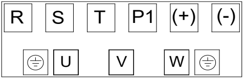
图 3-12 主回路端子图（三相 380V，90~1400kW）
