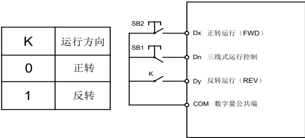
图 6-8 三线式控制模式 2
