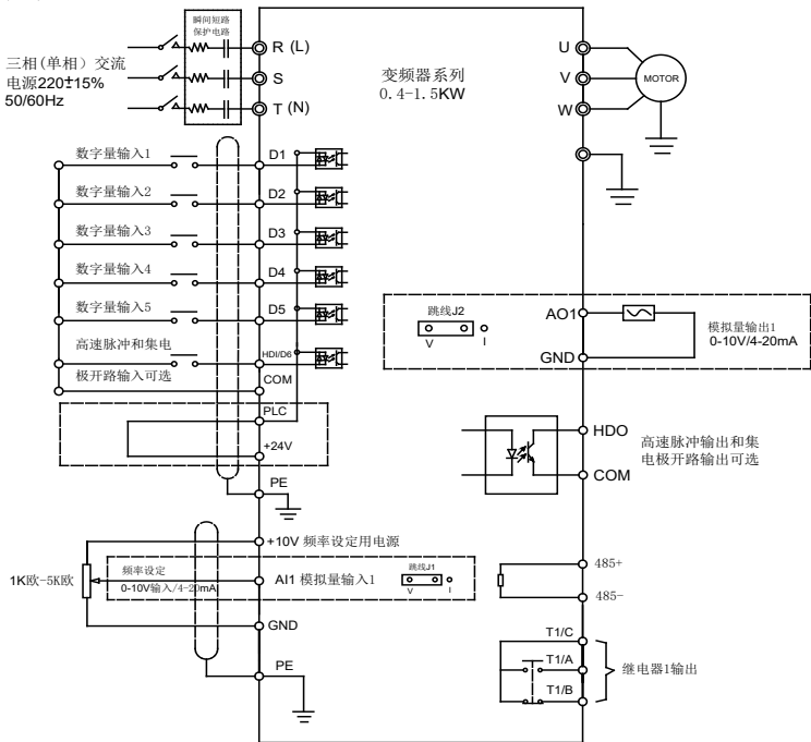
图 3-3 单相/三相 220V 0.4~1.5kW 变频器接线图
