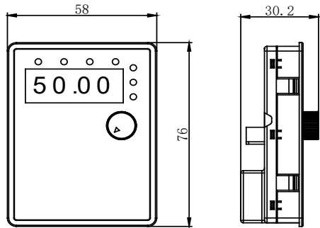
单相/三相 220V 0.4~1.5kW 变频器用 58*76mm 键盘尺寸(X 系列)
