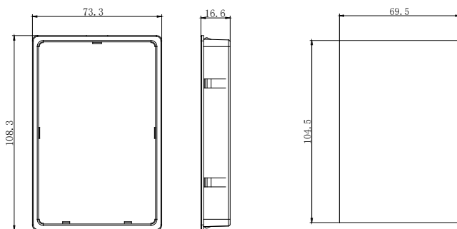
65*100mm 键盘托架尺寸
